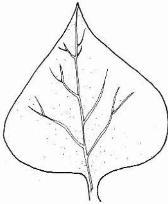
1 Deltate
