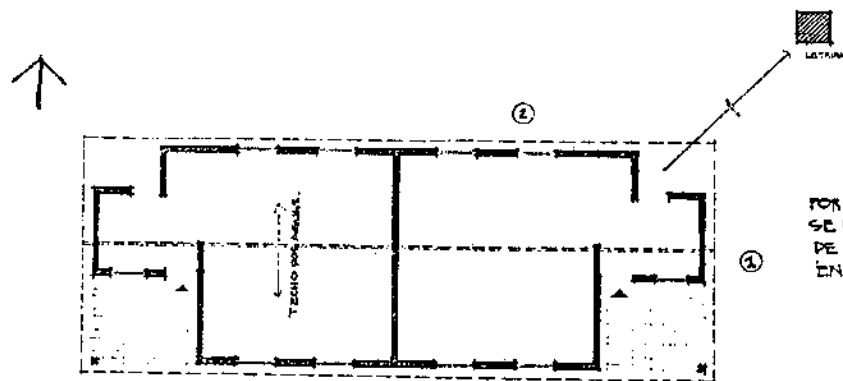
④ PLANTA CONJUNTO ESCALA 1:100
