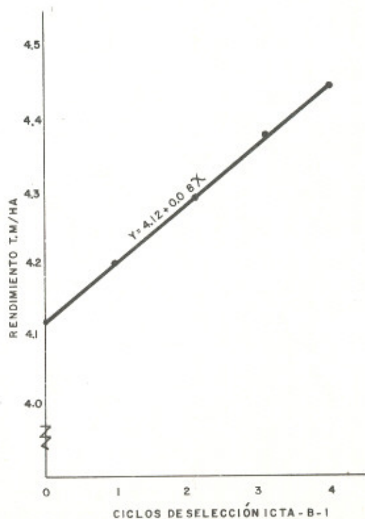
GRAFICA 1 LINEA DE REGRESIÓN PARA EL RENDIMIENTO EN EL ANALISIS COMBINADO EN LOS CICLOS DE SELECCIÓN DE ICTA B-1, 1976
