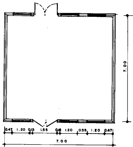
PLANTA GENERAL ESC. 1:100
