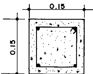
SECCION DE COLUMNA ESCALA 1=5
