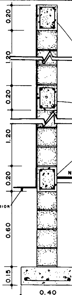
SECCION DE MURO ESC. 1=12.5
