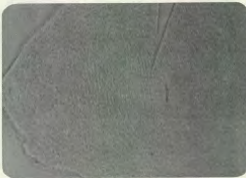
Figura 4. Corte fenestral de un quiste de H. (G) pallida , del grupo rostochiensis. (750 x)
