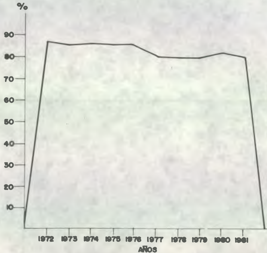
FIG. 14: DATOS DE HUMEDAD Y EVAPORACION, ULTIMOS 10 AÑOS REGION VALLE DEL POLOCHIC, ALTA VERAPAZ E IZABAL. AÑO 1982
