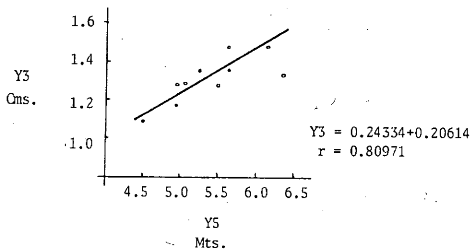
FIGURA 19. Bambusa multiplex . Curvas de correlación para las variables: longitud del 5to. entrenudo a partir del suelo (Y1), grosor de la pared del 5to. entrenudo a partir del suelo (Y2), diámetro del 5to. entrenudo a partir del suelo (Y3) y longitud del tallo. (Y5).
