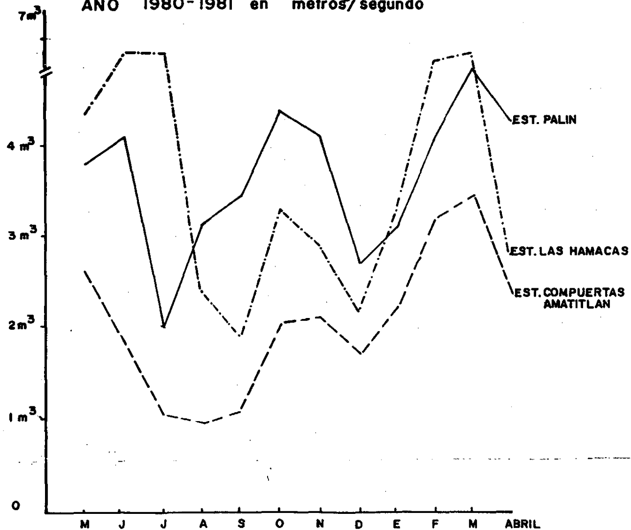
GRAFICA DE CAUDALES MEDIOS MENSUALES RIO MICHATOYA AÑO 1980-1981 en metros 3 /segundo
