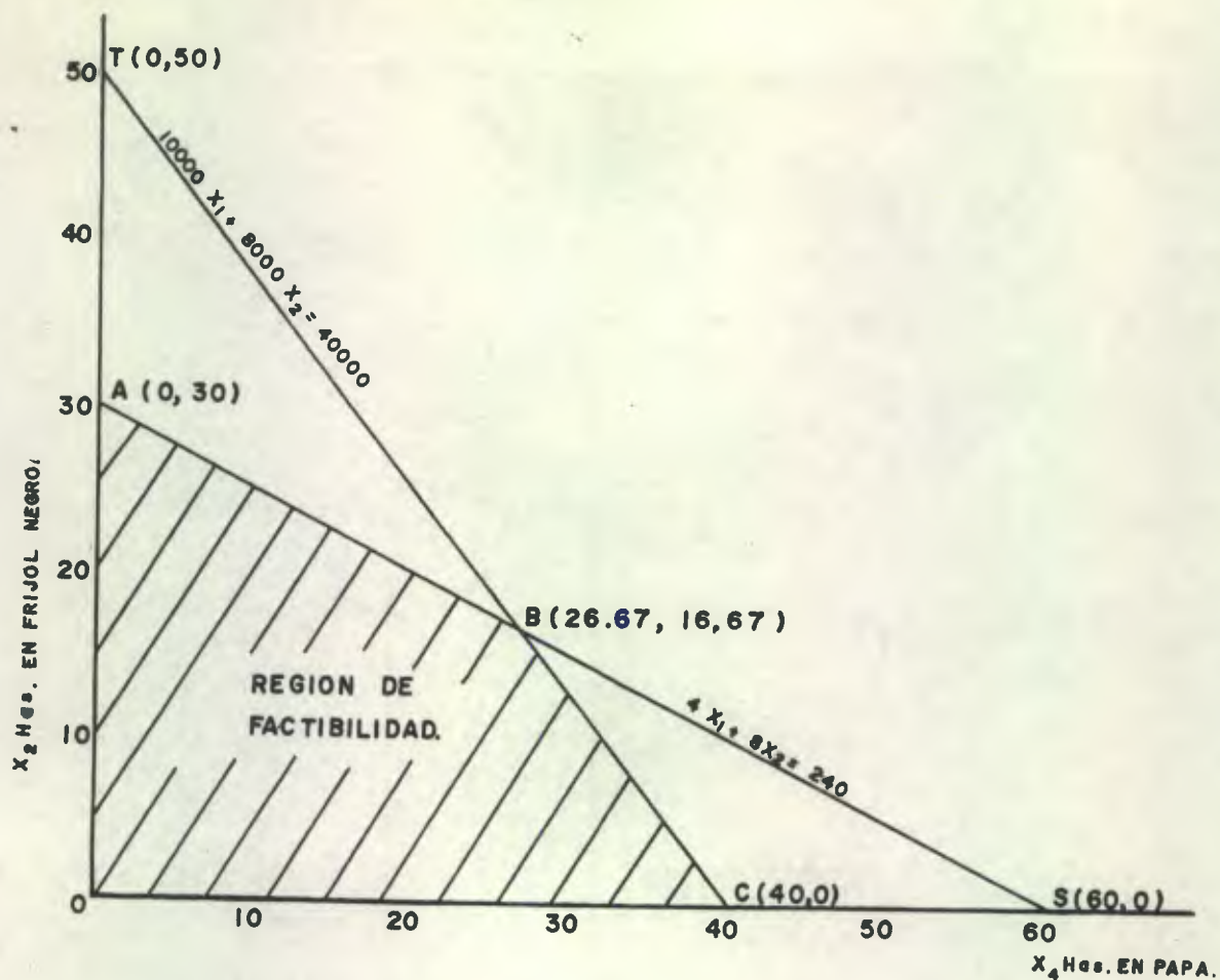
FIGURA 1. DETERMINACION DE LA REGION DE FACTIBILIDAD DEL PROBLEMA.
