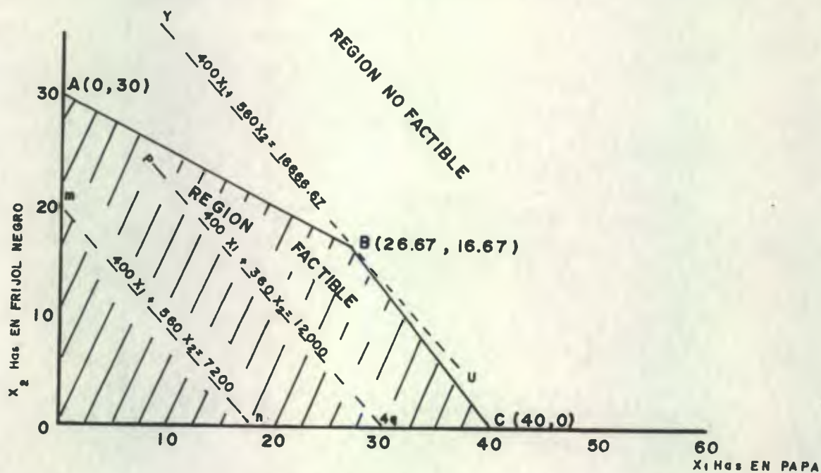
FIGURA 1. DETERMINACION DE LA REGION DE FACTIBILIDAD DEL PROBLEMA.
