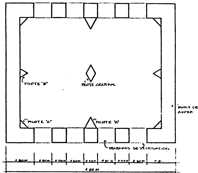
PLANTA ACOTADA
