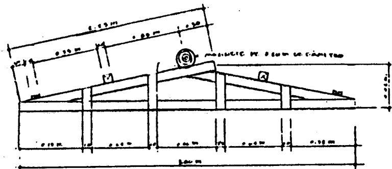
TIJERA ESCALA 1:20
