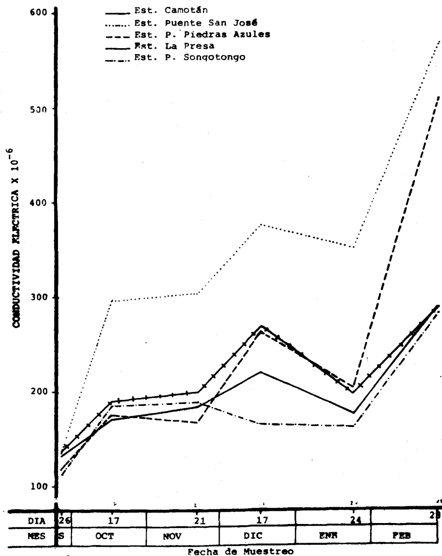
Fig. No. 6. Variación de la Conductividad Eléctrica en cinco estaciones de muestreo de agua superficial en la cuenca del Río Grande de Zacapa, durante el período Sep/83 a Feb/84.
