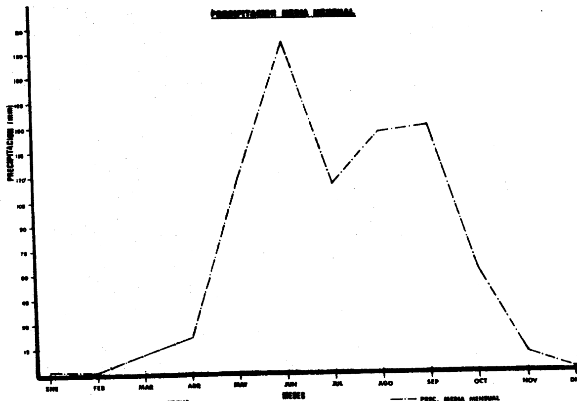
Fig. No. 20 Variación de la precipitación media mensual en la estación Chiquimula-Fequa
