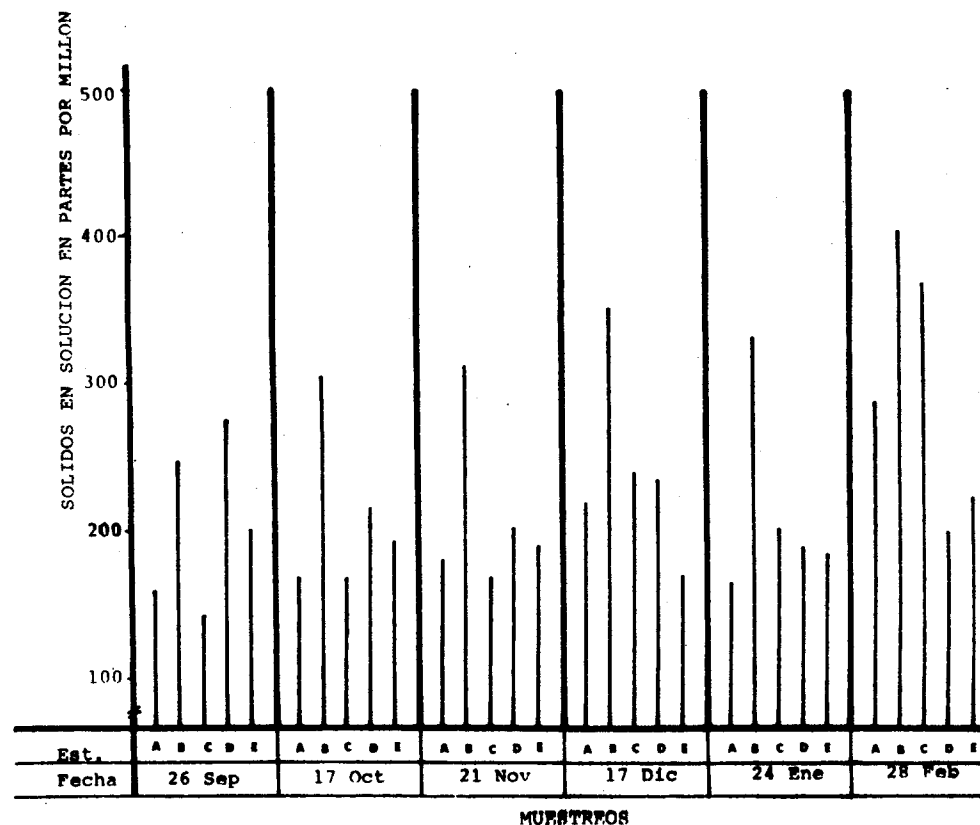
Figura No. 9. Valor de los sólidos en solución durante seis meses de muestreo de agua superficial en cinco estaciones en la cuenca del Río Grande de Zacapa, durante el período de Septiembre de 1983 a Febrero de 1984. - (A. Estación Camotán, B. Estación Puente San José, C. Estación Puente Piedras Azules, D. Estación La Presa, E. Estación Puente Songotongo).
