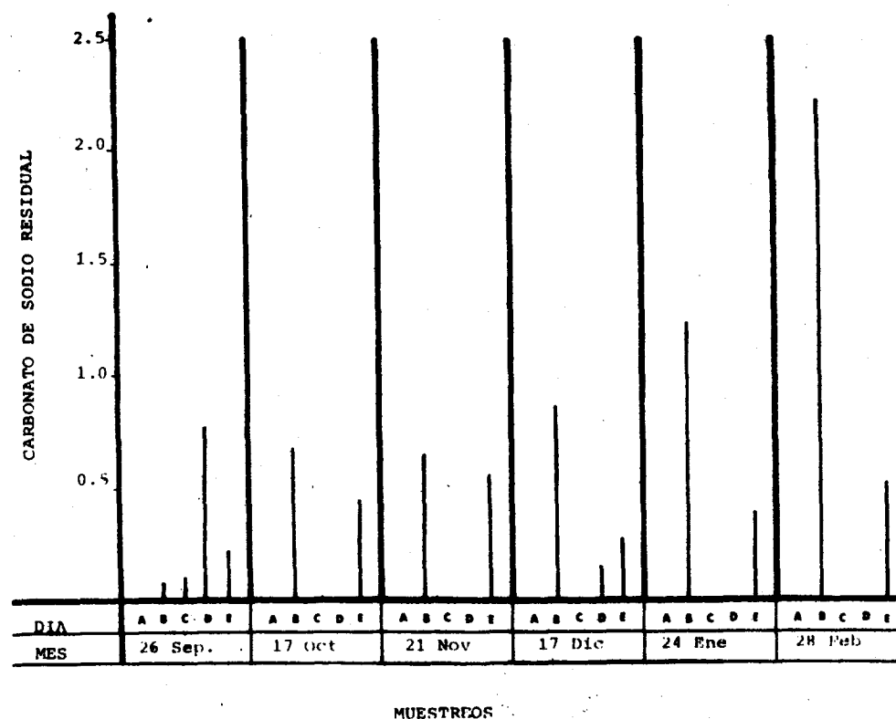
Figura No. 17. Valor de carbonato de sodio residual durante seis muestreos del agua superficial en cinco estaciones de muestreo en la cuenca del Río Grande de Zacapa, durante el período de Septiembre de 1983 a Febrero de 1984. (A. Estación Camotán, B. Estación Puente San José, C. Estación Puente Piedras Azules, D. Estación La Presa, E. Estación Puente Songopongo).
