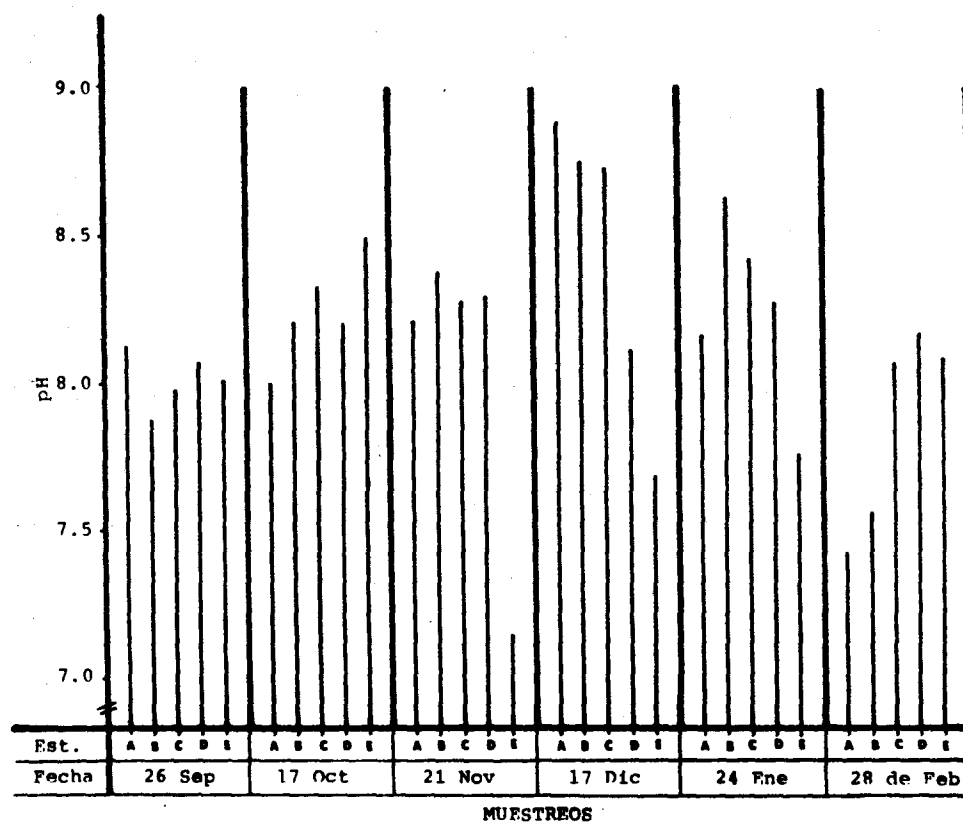
Figura No. 5. Valor de pH durante seis muestreos del agua superficial en cinco estaciones de muestreo en la cuenca del Río Grande de Zacapa durante el período de Septiembre de 1983 a Febrero de 1984. (A. Estación Camotán, B. Estación Puente San José, - C. Estación Puente Piedras Azules, D. Estación La Presa, E. Estación Puente Songotongo).
