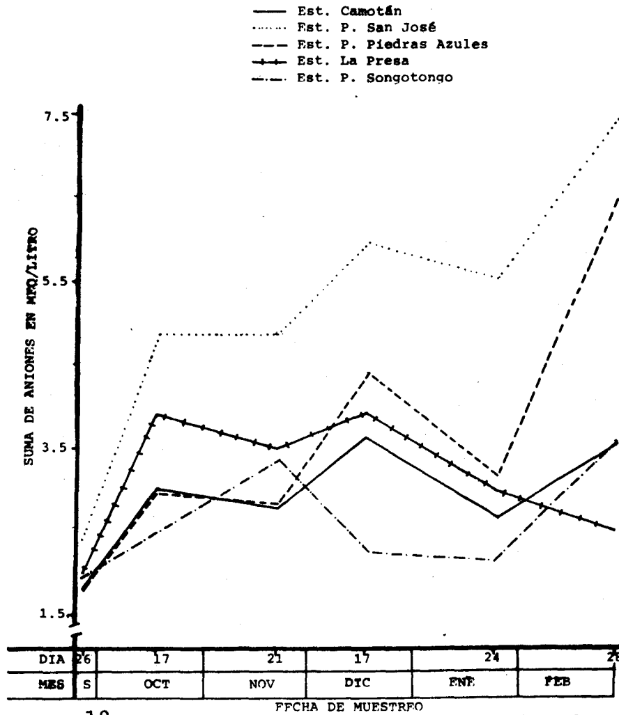
Fig. No. 12 Variación de la Suma de Aniones en cinco estaciones de muestreo de agua superficial en la cuenca del Río Grande de Zapaca, durante el período Sep/83 a Feb/84.
