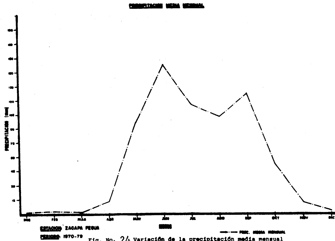
Fig. No. 24 Variación de la precipitación media mensual en la estación Zacapa-Peque.
