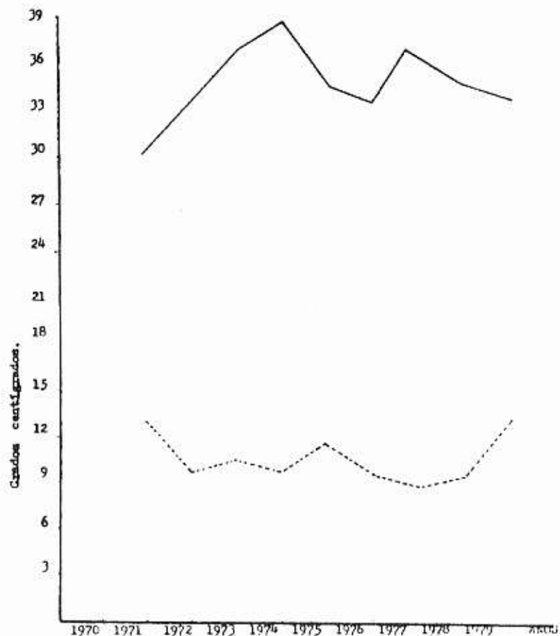
FIGURA No. 4 Temperaturas Máximas y Mínimas, últimos 10 años La Unión, Zacapa, 1984.
