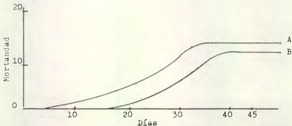
Gráfica - 9: Tendencia en la mortandad de dos poblaciones de Pachychilus sp. sometida a dos ambientes distintos: (A, agua tomada en el punto de desembocadura de la escorrentía de la fosa de lodos del pozo San Román II y B, agua tomada 100 metros aguas arriba del punto anterior), muestra tomada el 20-4-84.
