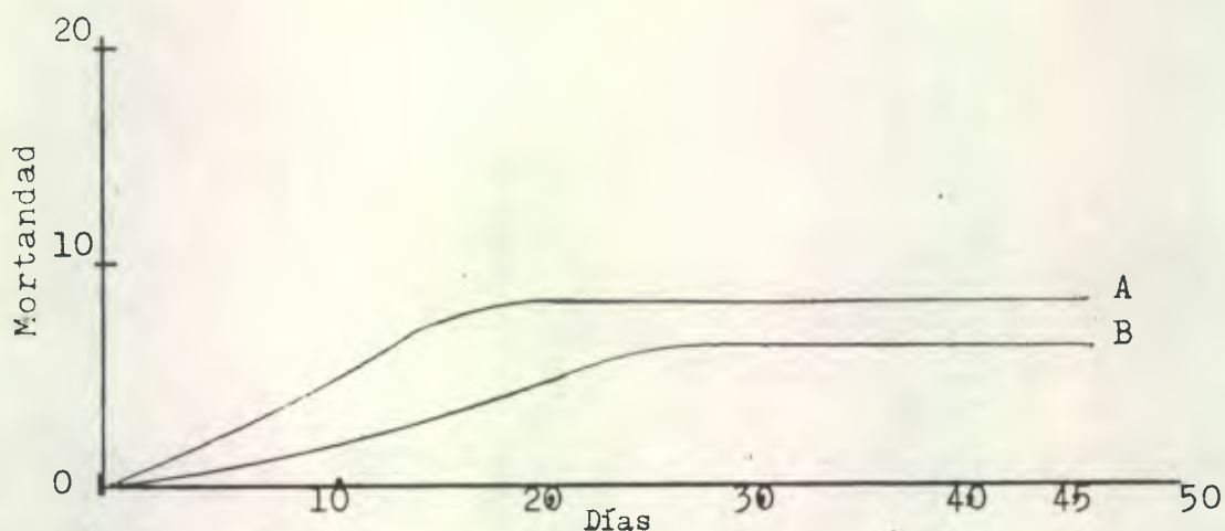
Gráfica - 8: Tendencia en la mortandad de dos poblaciones de Tilapia sp. sometidas a dos ambientes distintos: (A, agua tomada en el punto de desembocadura de la escorrentía de la fosa de lodos del pozo San Román II y B, agua tomada 100 metros aguas arriba del punto anterior), muestra tomada el 20-4-84.
