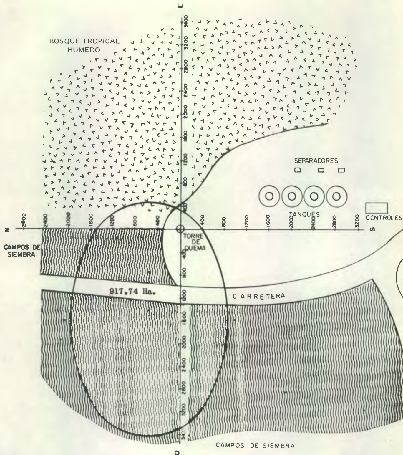
Gráfica - 11: Area Mínima afectada por la acción fitotóxica de los aeropoluantes.
