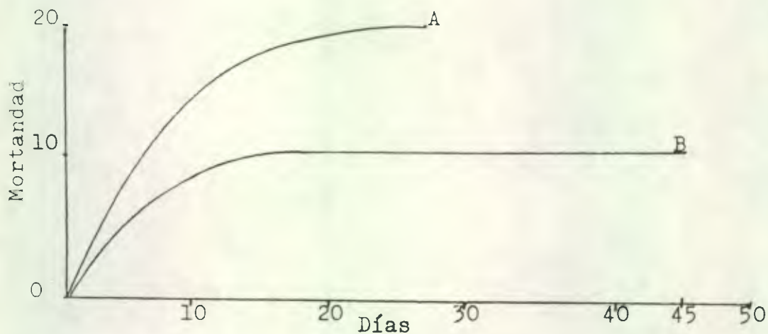
Gráfica - 7: Tendencia en la mortandad de dos poblaciones de Potomocarcinus guatemalensis . Sometidas a dos ambientes distintos; (A, agua tomada en el punto de desembocadura de la escorrentía de la fosa de lodos del pozo San Román II y B, agua tomada 100 metros aguas arriba del punto anterior), muestra tomada el 19-7-84.
