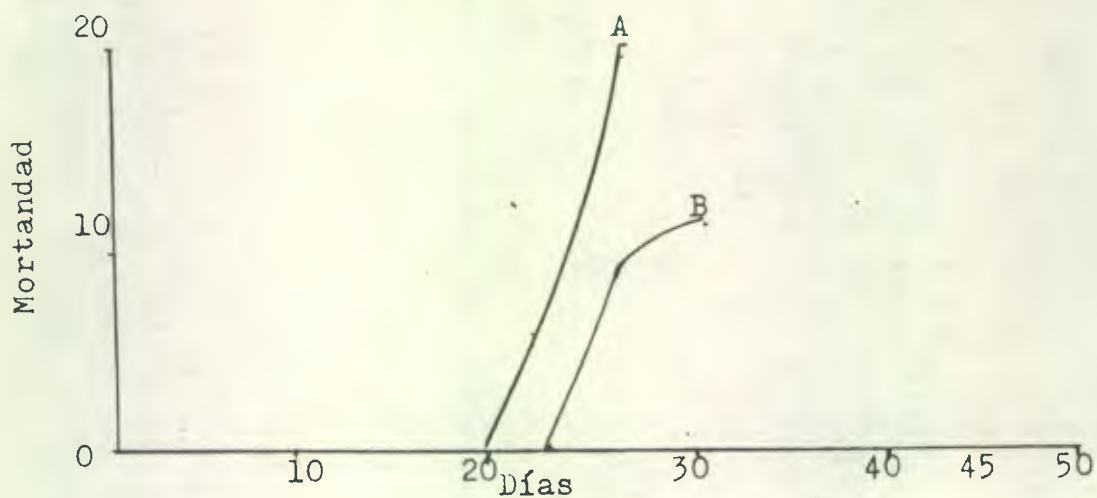
Gráfica - 4: Tendencia en la mortandad de dos poblaciones de Tilapia sp. sometidas a dos ambientes distintos; (A, agua tomada en el punto de desembocadura de la escorrentía de la fosa de lodos del pozo San Román II y B, agua tomada 100 metros aguas arriba del punto anterior), muestra tomada el 2-1-84.
