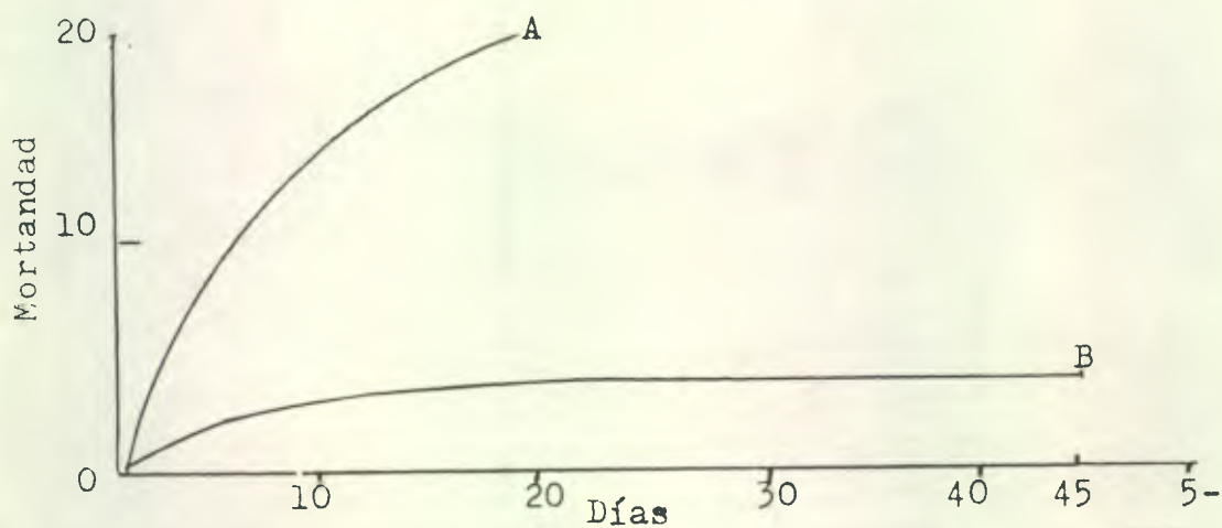
Gráfica - 4: Tendencia en la mortandad de dos poblaciones de Tilapia sp. sometidas a dos ambientes distintos; (A, agua tomada en el punto de desembocadura de la escorrentía de la fosa de lodos del pozo San Román II y B, agua tomada 100 metros aguas arriba del punto anterior), muestra tomada el 2-1-84.
