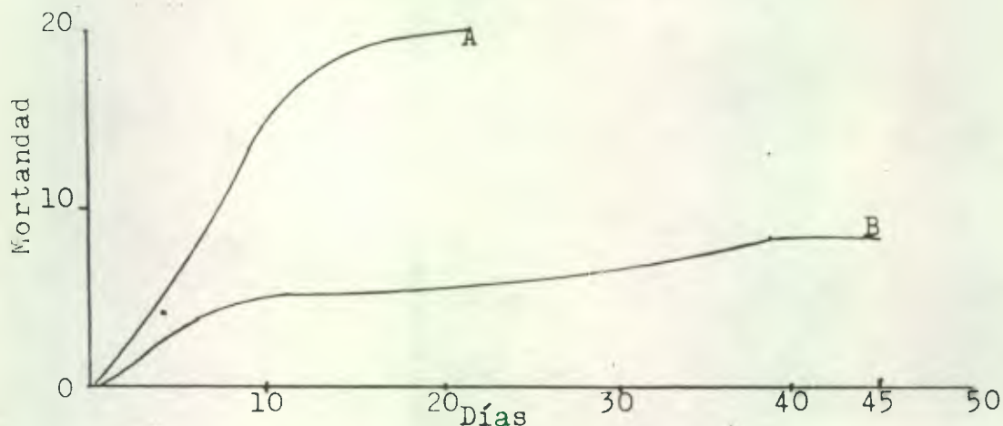
Gráfica-6: Tendencia en la mortandad de dos poblaciones de Pachychilus sp. sometidas a dos ambientes distintos; (A, agua tomada en el punto de desembocadura de la escorrentía de la fosa de lodos del pozo San Román II y B, agua tomada 100 metros aguas arriba del punto anterior), muestra tomada el 19-7-84.
