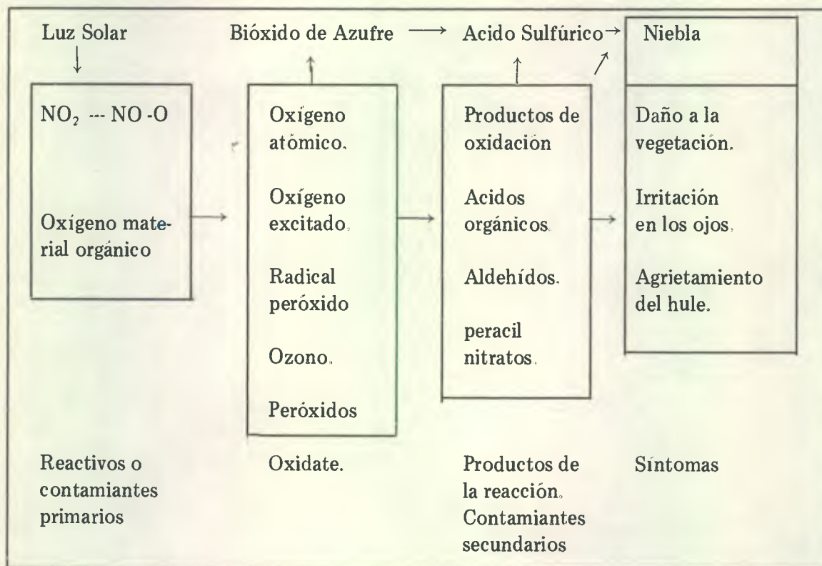
Gráfica 2: Reacciones fotoquímicas que se presentan en el smog fotoquímico. (Tomada de Sutton y Harmón (11).
