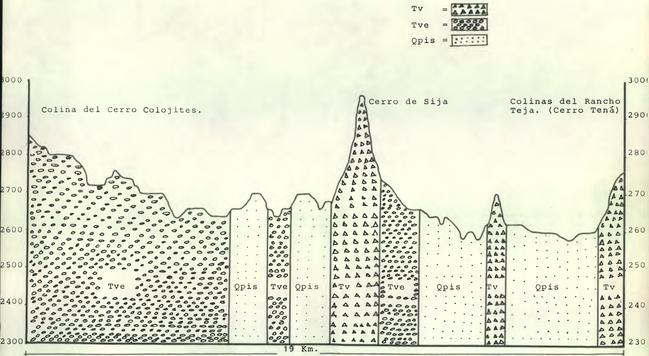
FIGURA 6. PERFIL TRANSVERSAL DE LA CUENCA DEL RIO SAMALA (FASE I), DE LOS MUNICIPIOS DE SIBILIA A LA ALDEA RANCHO DE TEJA.
