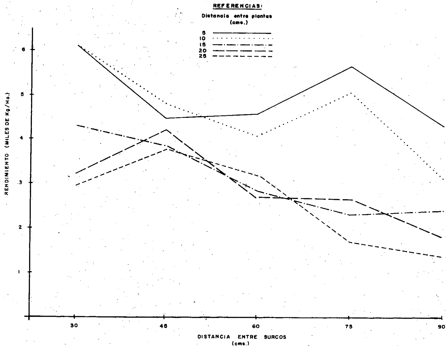
FIGURA No. 2 Respuesta del Sorgo ICTA-450 a la interacción de la distancia entre surcos y plantas. Localidad: GUAZACAPAN, SANTA ROSA, 1984
