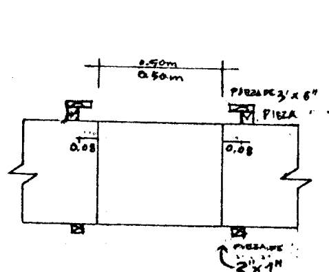
DETALLE EN PLANTA DE VENTANA DE VENTILACION
