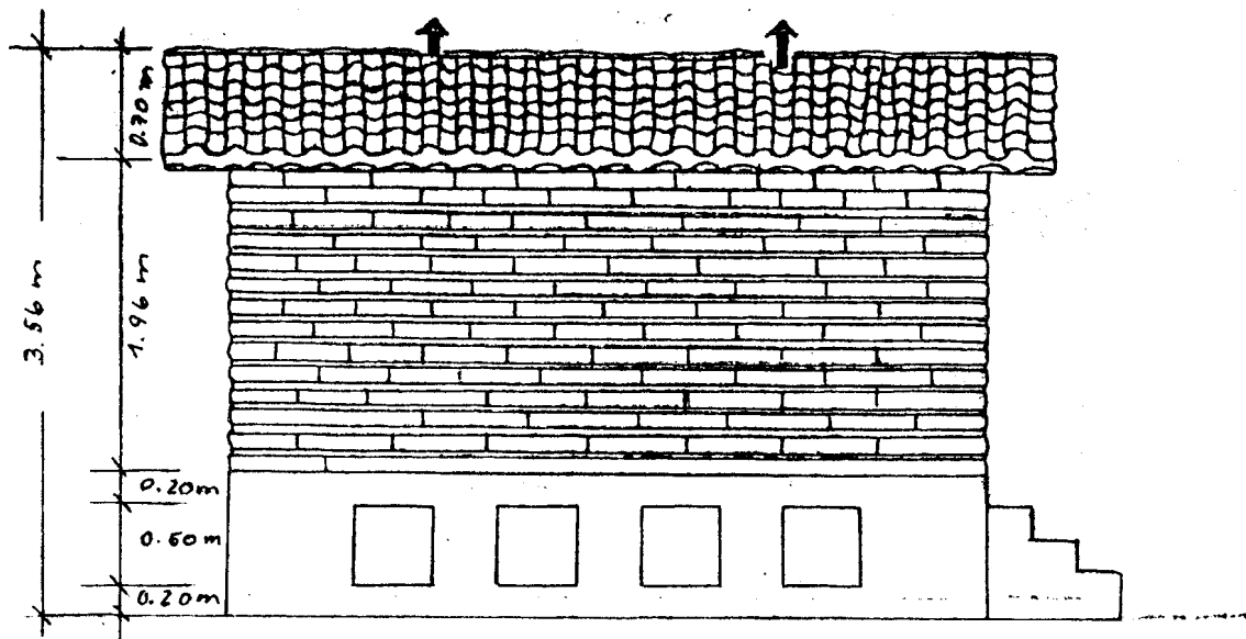
ELEVACION LATERAL
