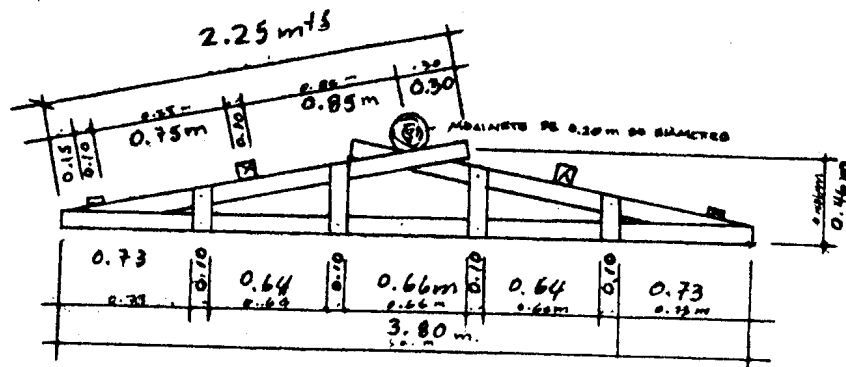
TIJERA ESCALA 1:20
