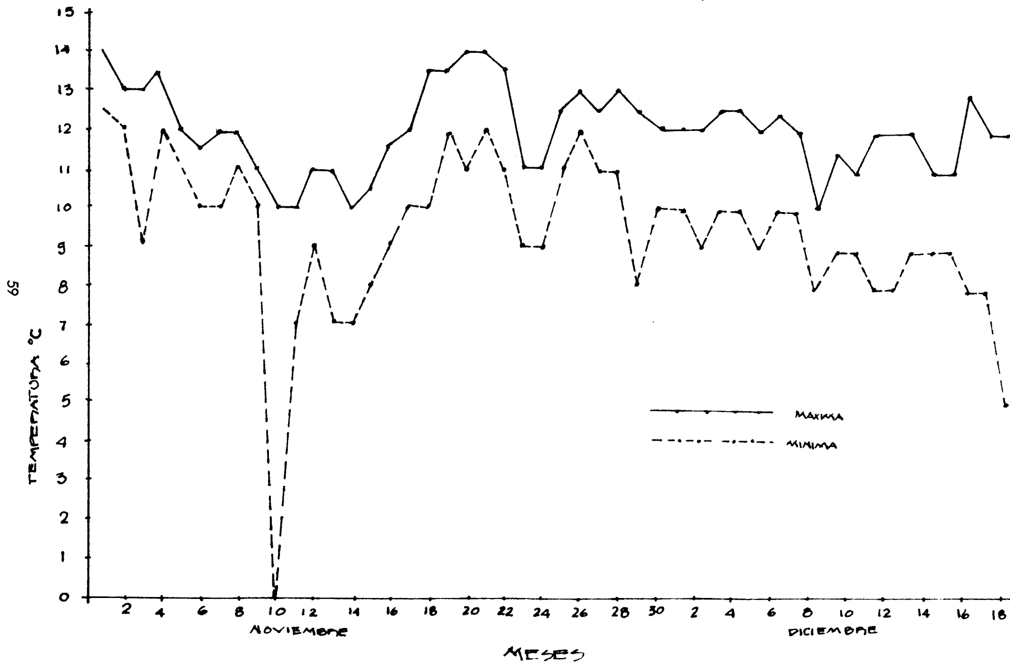
GRAFICA No. 2 Temperaturas máximas y mínimas registradas durante el tiempo de almacenamiento. Meses noviembre y diciembre.
