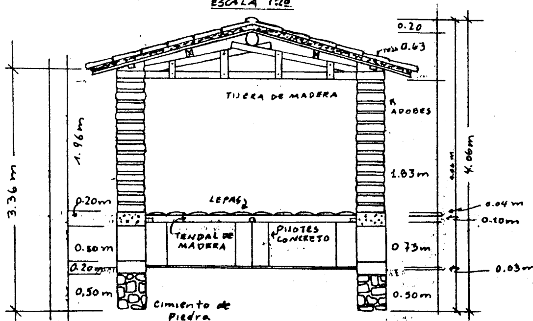
CORTE A-A
