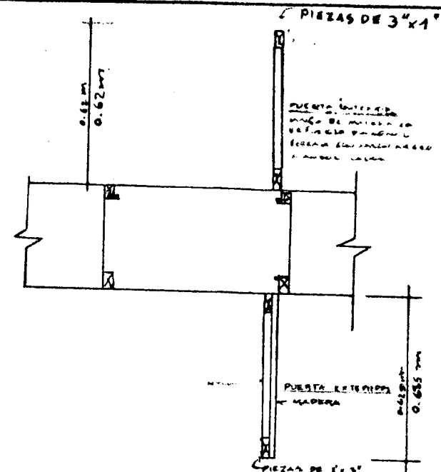
DETALLE EN PLANTA DE PUERTA
