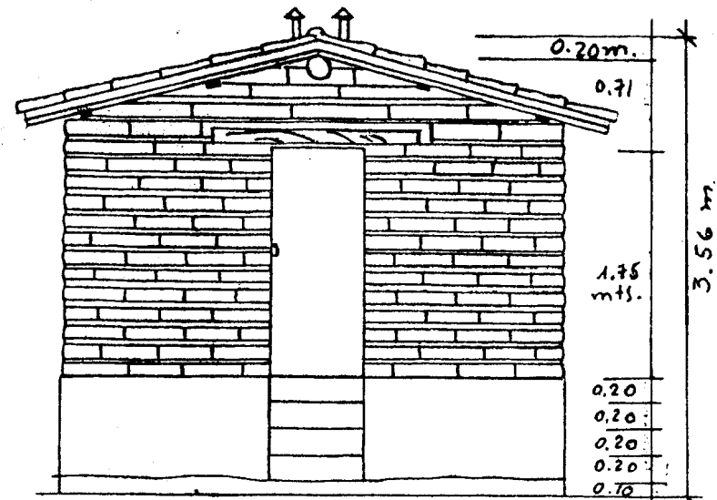
ELEVACION FRONTAL
