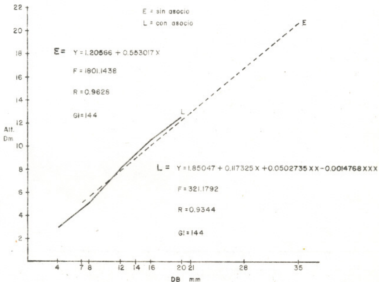
Fig. 20 Regresion Alt. (Dm)/DB(mm) Grevillea robusta con asocio y sin asocio
