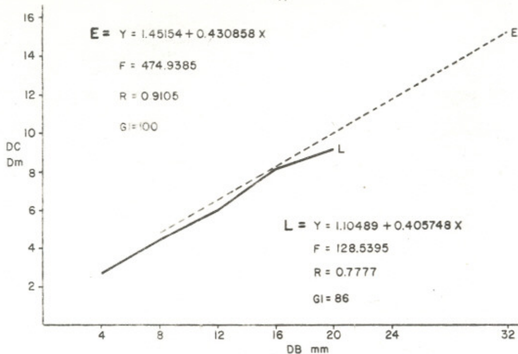
Fig. 15 Regresión DC(Dm)/DB(mm) Eucalyptus citriodora procedencia Guatemala sin asocio y con asocio
