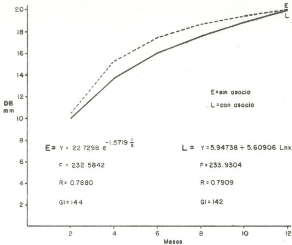
Fig. 21 Regresión DB (mm)/Edad en meses Alnus acuminata sin asocio y con asocio.
