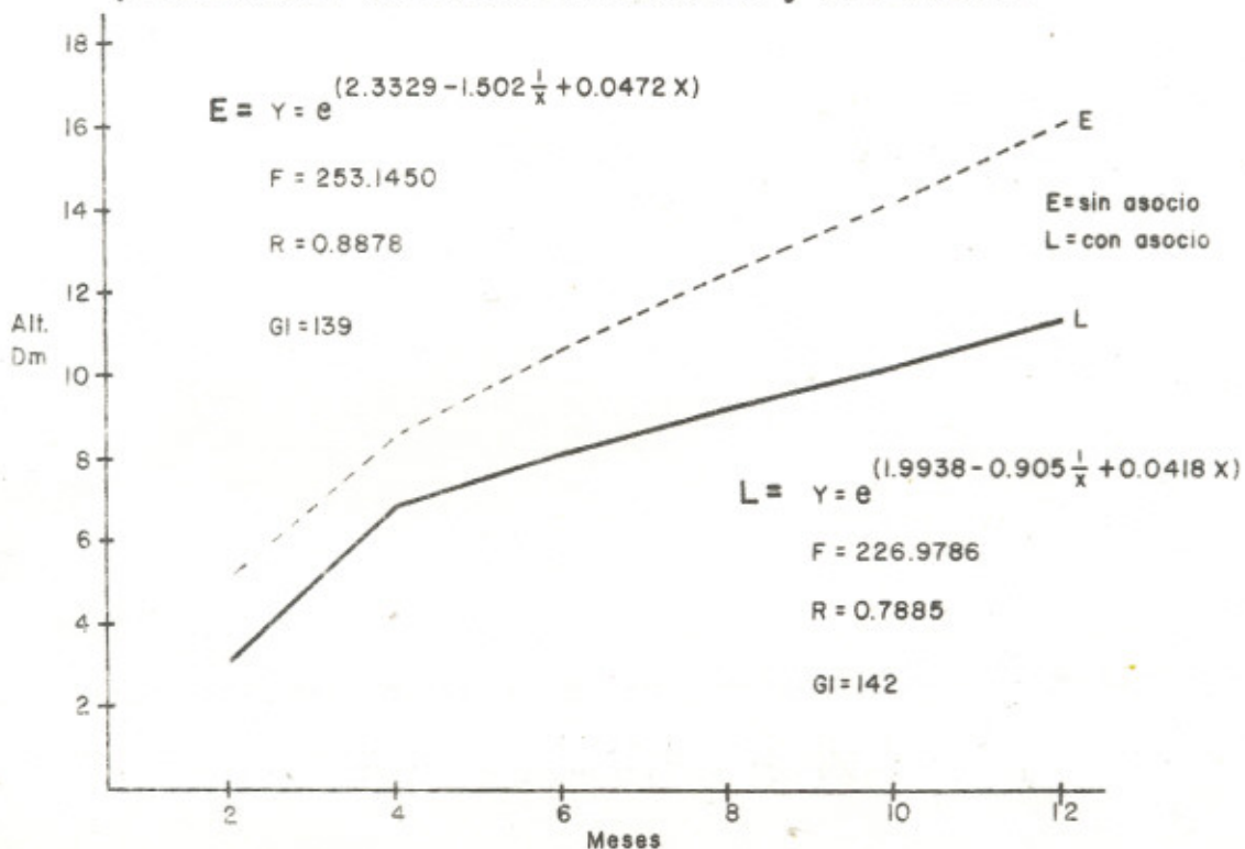
Fig. 14 Regresión Alt. (Dm)/Edad en meses Eucalyptus citriodora procedencia Guatemala sin asocio y con asocio.
