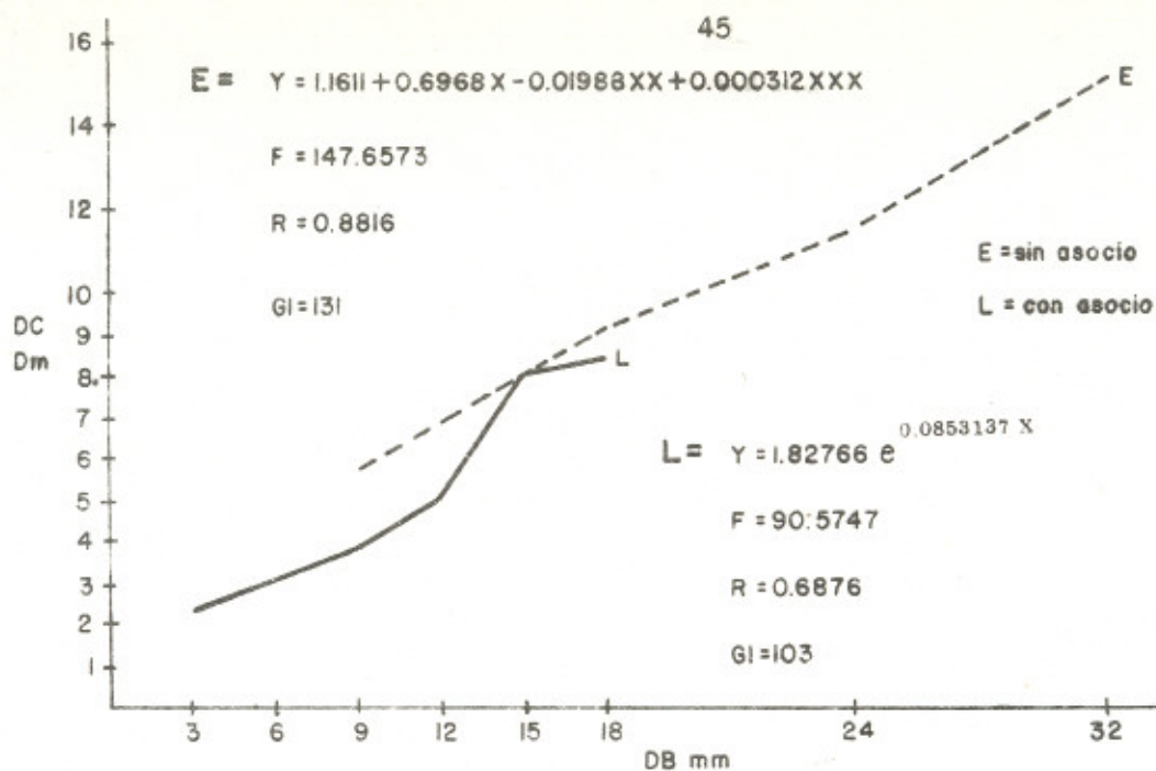
Fig. 11 Regresión DC(Dm)/DB(mm) Eucalyptus citriodora procedencia Brasil sin asocio y con asocio.
