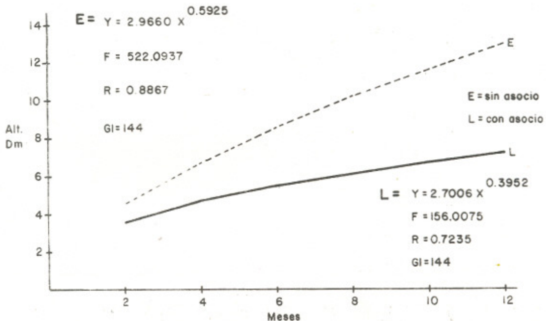
Fig. 18 Regresión Alt. (Dm)/Edad en meses Grevillea robusta sin asocio y con asocio.
