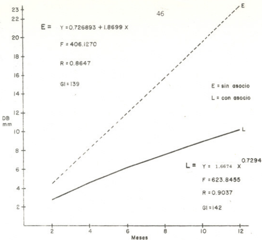
Fig. 13 Regresión DB(mm)/Edad en meses Eucalyptus citriodora procedencia Guatemala sin asocio y con asocio.
