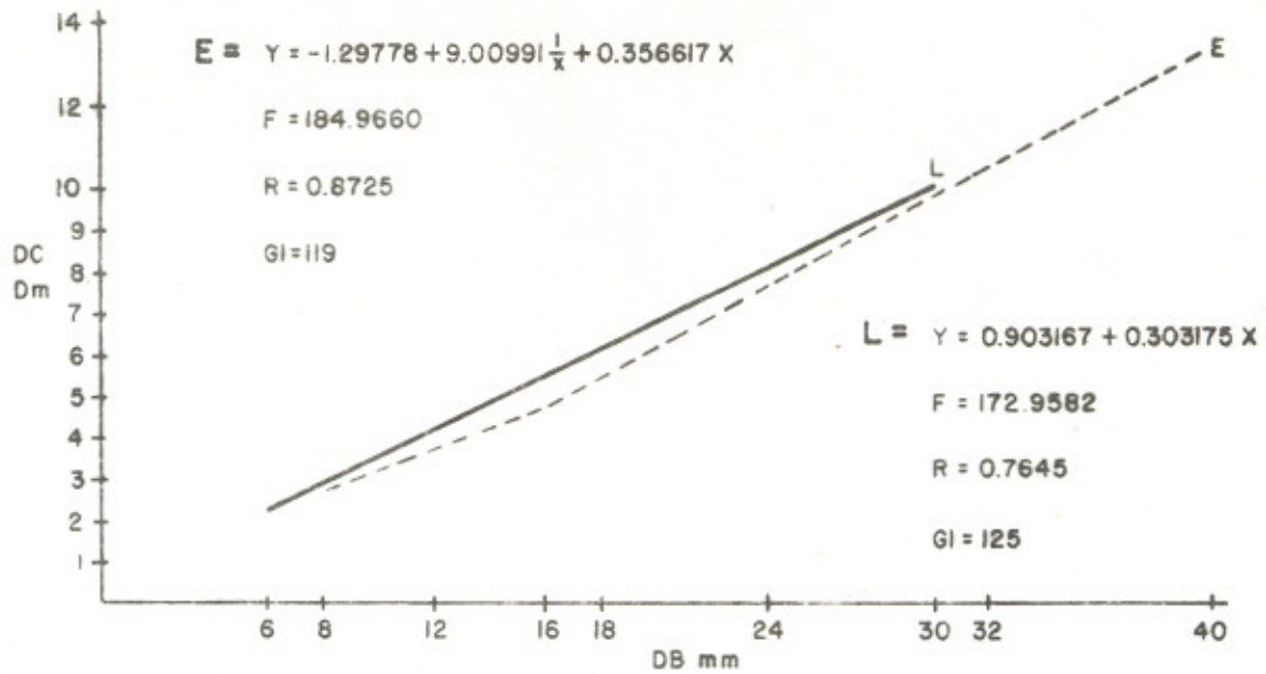
Fig. 23 Regresion DC (Dm)/DB (mm) Alnus acuminata con asocio y sin asocio
