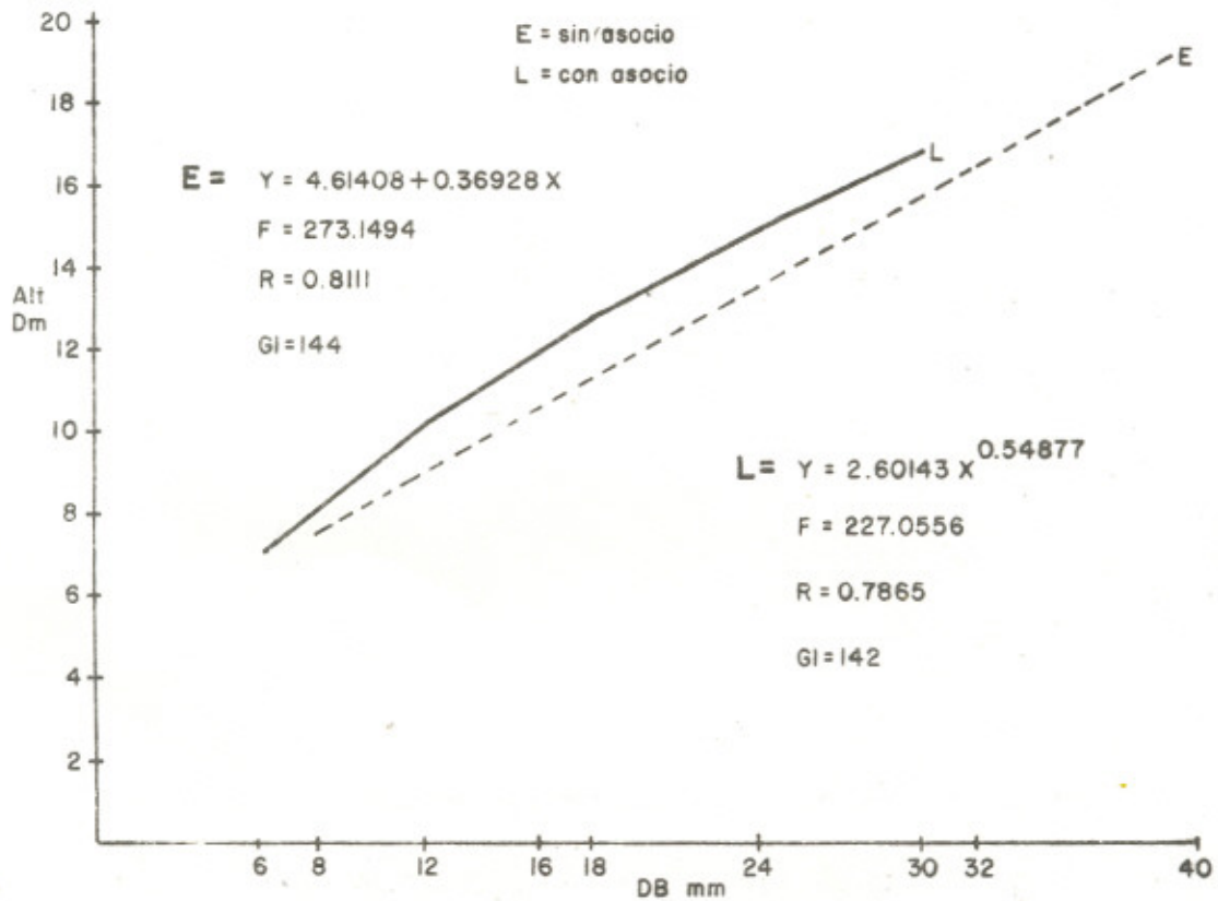
Fig. 24 Regresion Alt. (Dm)/DB (mm) Alnus acuminata con asocio y sin asocio
