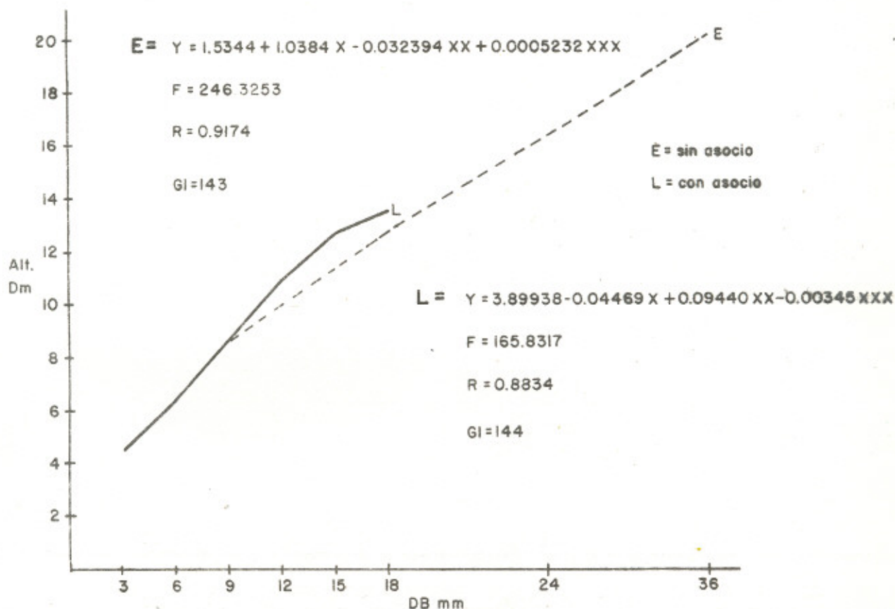
Fig. 12 Regresión Alt. (Dm)/DB(mm) Eucalyptus citriodora procedencia Brasil sin asocio y con asocio.
