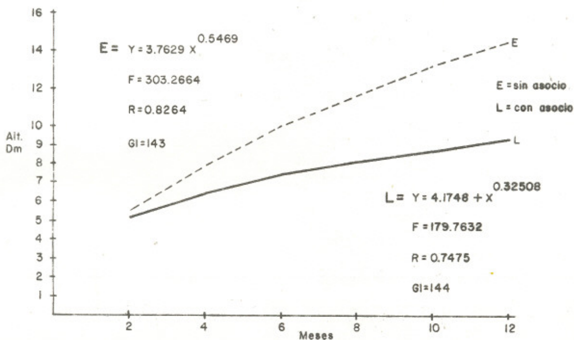
Fig. 10 Regresión Alt. (Dm)/Edad en meses Eucalyptus citriodora procedencia Brasil sin asocio y con asocio.
