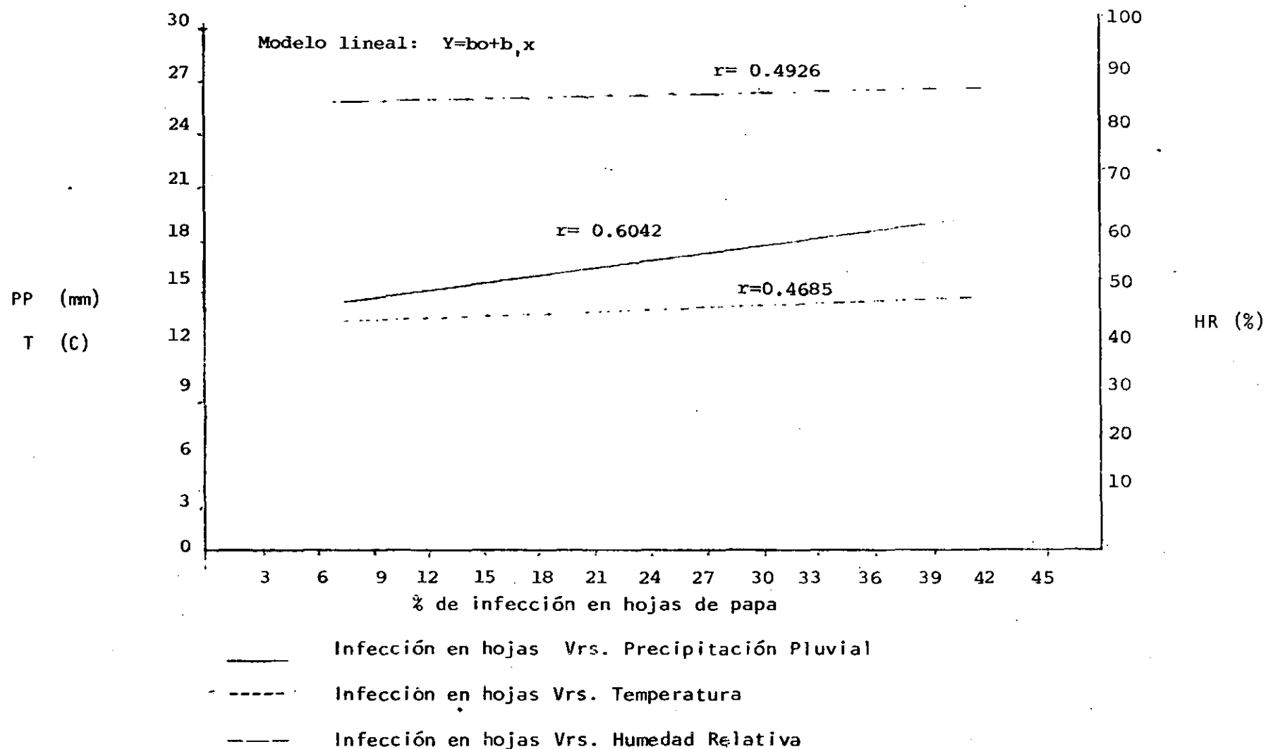
Gráfica No. 9: Comportamiento de P. infestans de acuerdo a condiciones climáticas y porcentaje de infección en hojas de papa durante el ciclo del cultivo en la localidad de Tecpán G.
