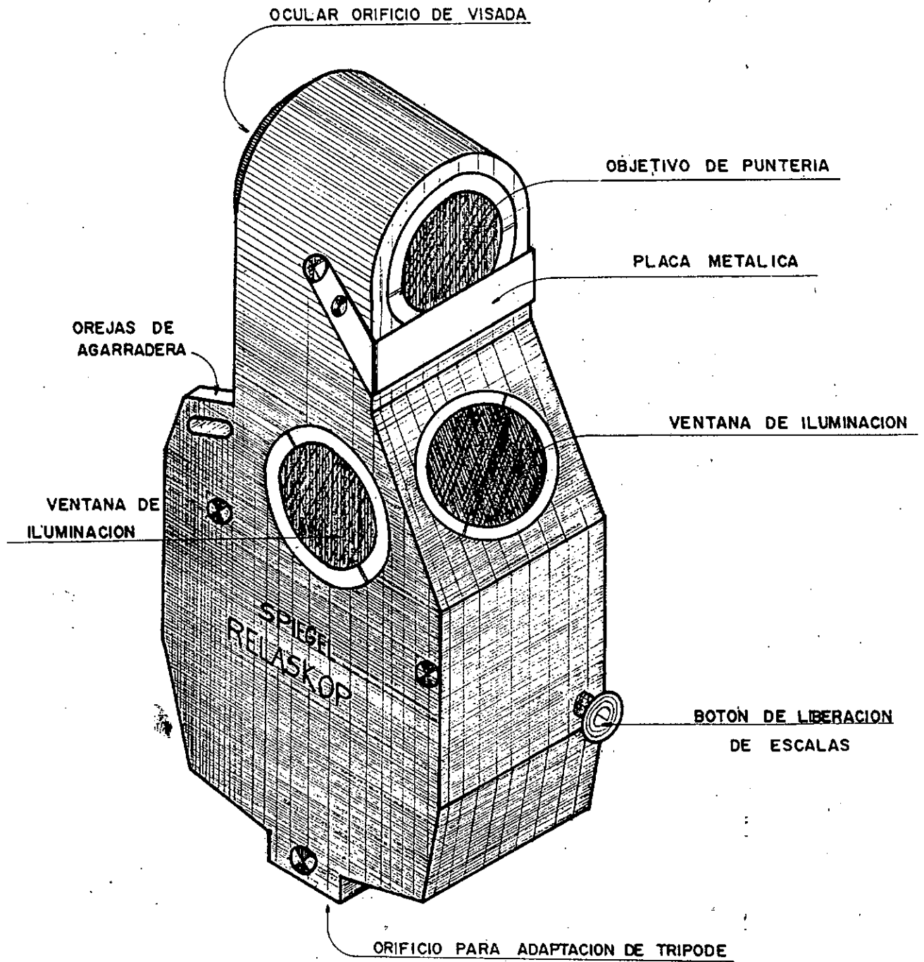
FIGURA 4 Relascopio de Bitterlich Escala Natural.
