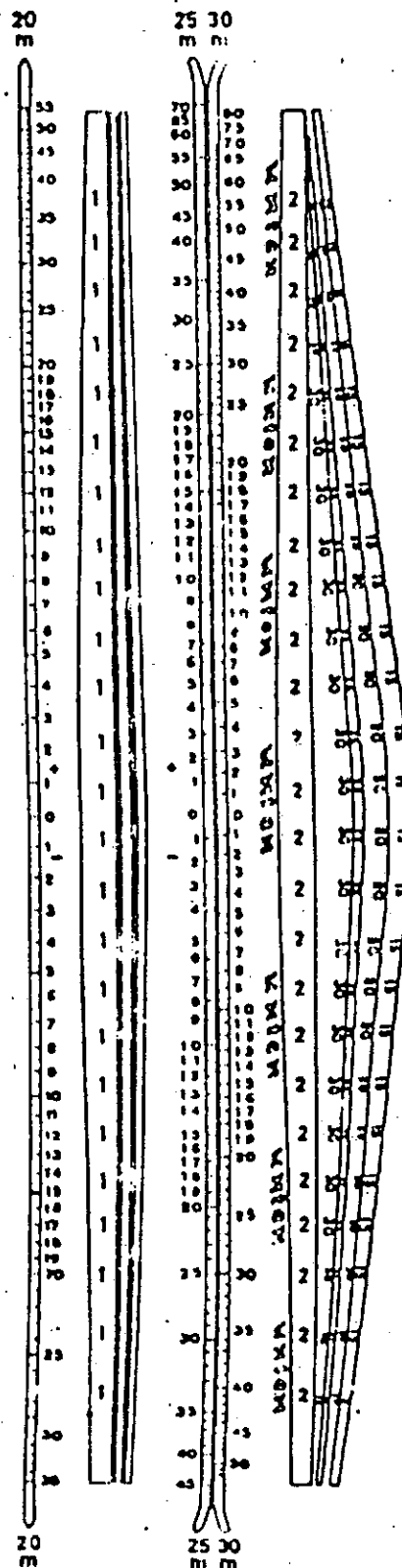
Figura 5. Bandas del Relascope de Bitterlich
