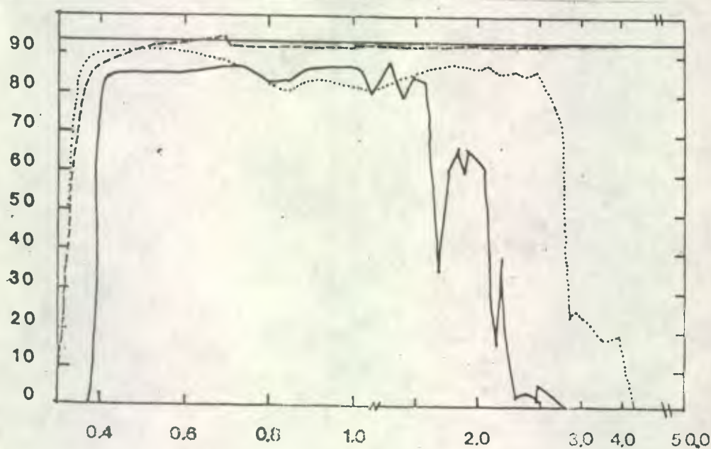
GRAFICA No. 8 TRANSMITIVIDAD DE RADIACION SOLAR (%) PARA ALGUNOS MATERIALES USADOS COMO CUBIERTAS DE COLECTORES PLANOS
