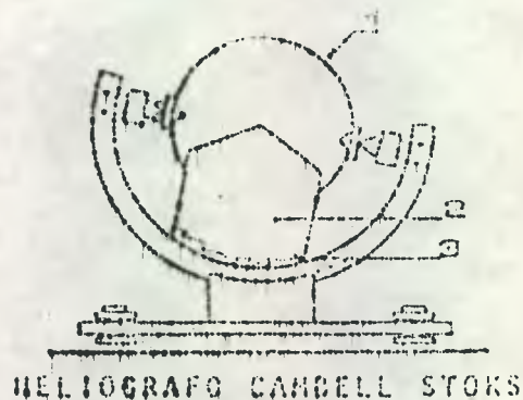
FIGURA No. 19 Equipo para medición de la radiación solar.
