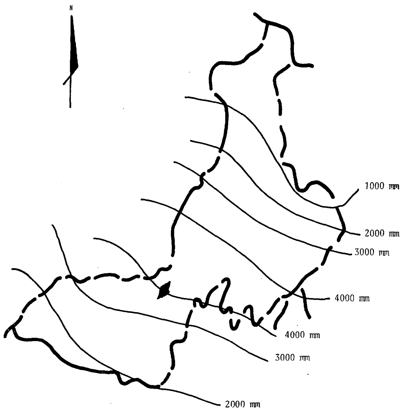
Fig. 2 Precipitación anual para el Dento. de Quezaltenango. Instituto de Sismología, Vulcanología, Meteorología e Hidrología (INSIVUMEH) Escala: 1:500,000
